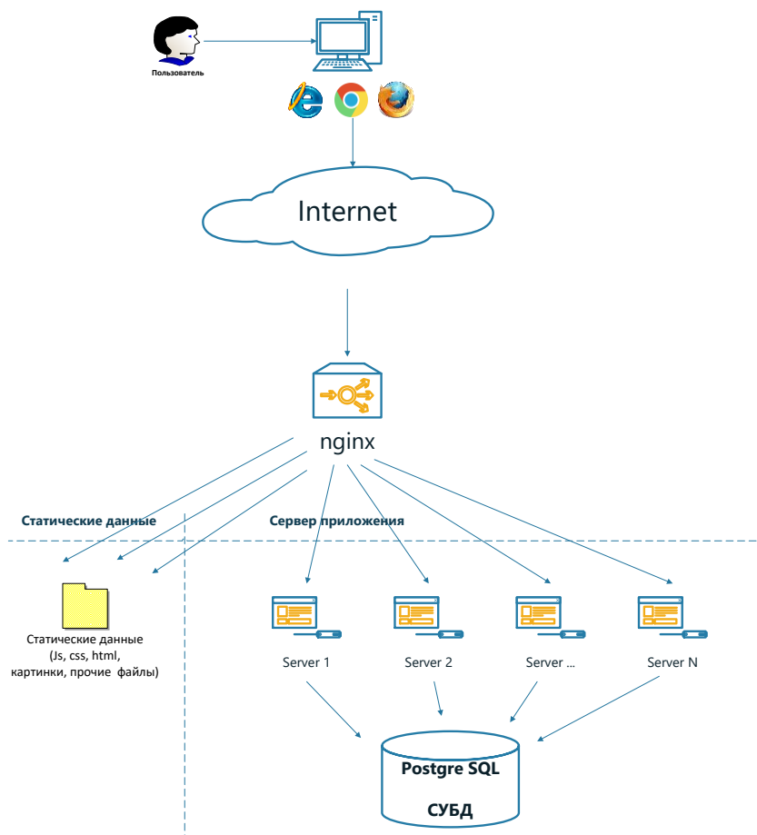
Рисунок 1 – Технологическая схема
